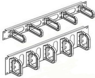
Panel de gestión de cables de 19"/1U y 19"/2U con 5 soportes
