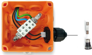
Elemento fusible adicional M25/2A
