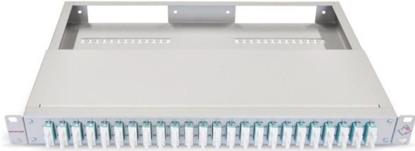
Compact voormonteerd paneel, 19"/1U, uitvoering met 8 MTP koppelingen (achteraan) en 48 OM3 LCD poorten in het turkoois (vooraan)
