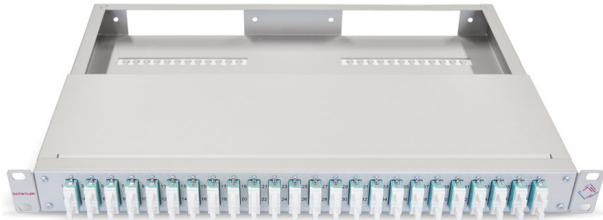
Kompaktes, vorkonfektioniertes 19"/1HE-Panel, Ausführungsbeispiel mit 8 MTP-Kupplungen (rückseitig) und 48 LCD-Ports OM3 türkis (frontseitig)
