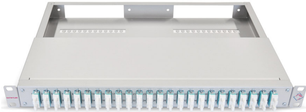
Panneau prémonté compact, 19"/1U, version avec 8 coupleurs MTP (face arrière) et 48 ports LCD OM3 en turquoise (face avant)
