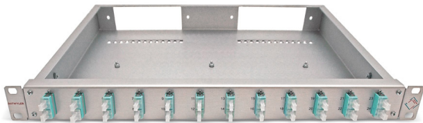
Kompaktes 19"/1HE-Breakout-Panel, Ausführung mit 12 LCQ-Ports, OM3 türkis
