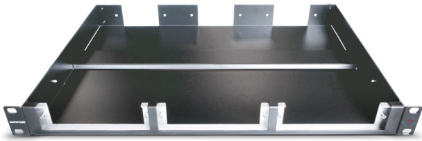
Panneau FO-DCS 19"/1U, equipable de manière modulaire
