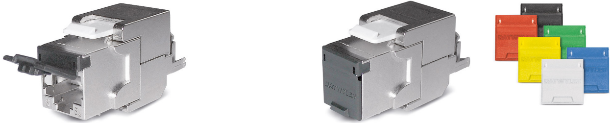
RJ45-Modul KS-T 1/8 toolless Cat. 6/EA, mit Staubschutzklappe
