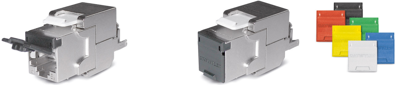
RJ45 module KS-T 1/8 tool-less Cat.6/E A met stofluikje
