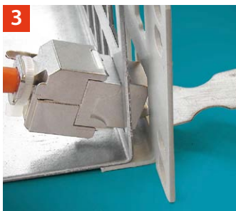
3 Modul schräg einsetzen Insert the jack obliquely
