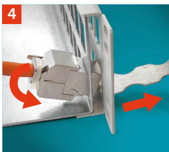
4 Modul nach unten in die Öffnung einkippen; dabei das Montage-Tool nach vorne ziehen Insert the jack completely while pulling the mounting tool at the same time.
