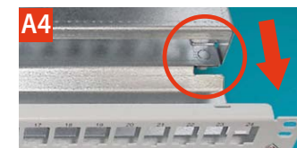
A4 Obere Kabelabfangung nach vorne (Richtung Frontplatte) schieben Push the upper cable strain relief forward (towards the front plate)
