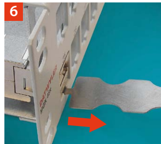
6 Montage-Tool noch vorne herausziehen, bis die Feder unter dem Modul einschnappt Pull out the mounting tool until the spring (on the bottom of the jack) snaps in
